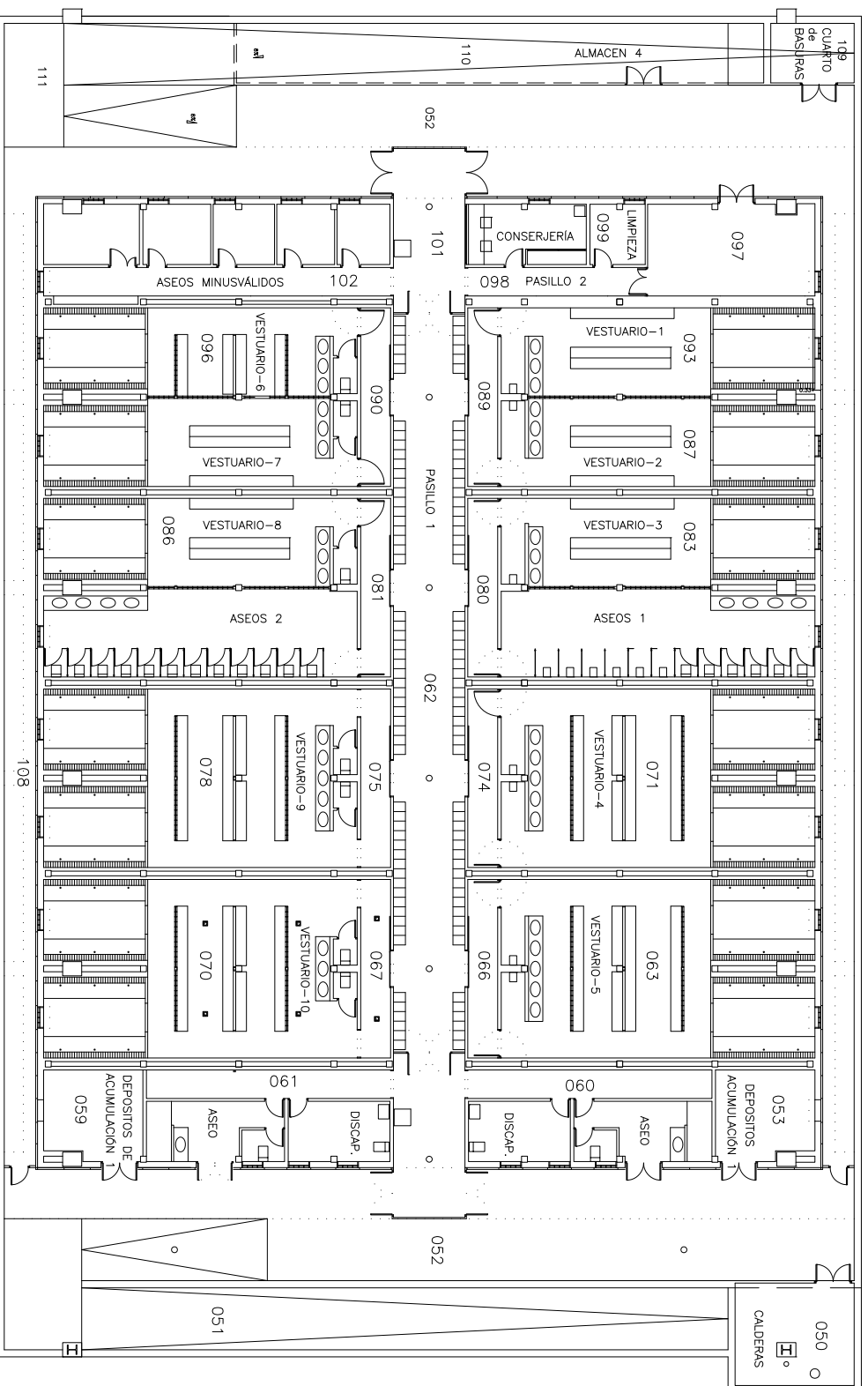
PLANTA SÓTANO.
